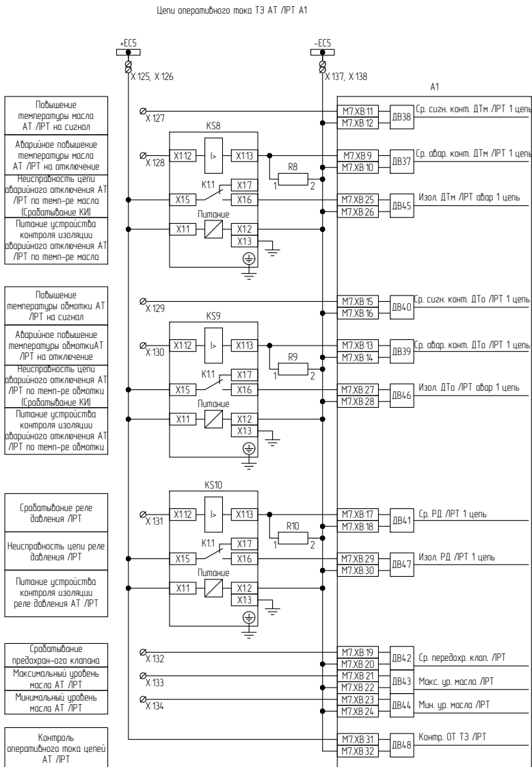
Рисунок Г.5 – Схема электрическая принципиальная (часть 5)
